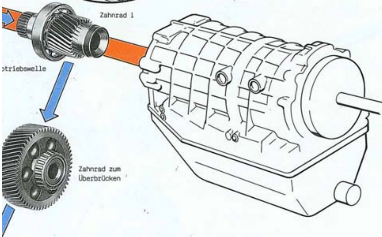
Lamellenkupplung mit Sperrfunktion
